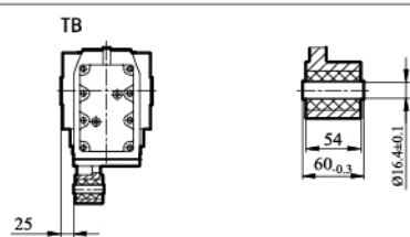
KV/ KVZ/ KVF67输出轴
