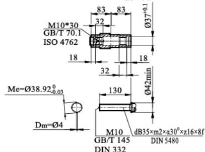
KV / KVZ / KVF57输出轴
