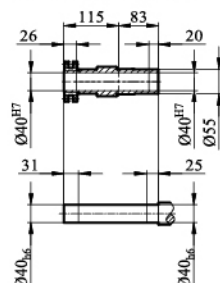
KH / KHZ / KHF57输出轴
