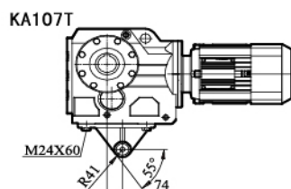
KA/ KAZ/ KAF107输出轴
