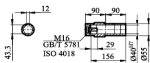
KA/ KAZ/ KAF67输出轴
