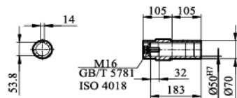
KA/ KAZ/ KAF77输出轴
