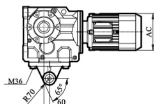
KA/ KAZ/ KAF127输出轴
