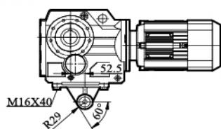
KA/ KAZ/ KAF77输出轴
