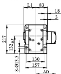
KA57B / KH57B / KV57B
