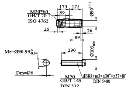
KV/ KVZ/ KVF107输出轴
