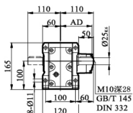
KA/ KH/ KV37
