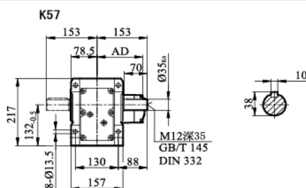
KA / KH / KV57
