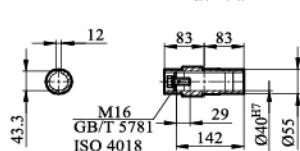
KA / KAZ / KAF57输出轴
