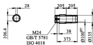
KA/ KAZ/ KAF127输出轴
