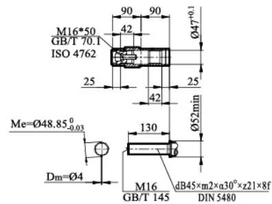
KV/ KVZ/ KVF67输出轴
