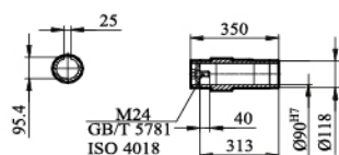
KA/ KAZ/ KAF107输出轴
