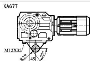
KA/ KAZ/ KAF67输出轴
