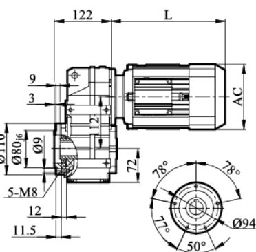
FAF/ FHF/ FVF37
