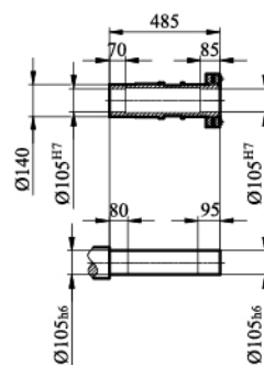
FH/ FHZ/ FHF127输出轴
