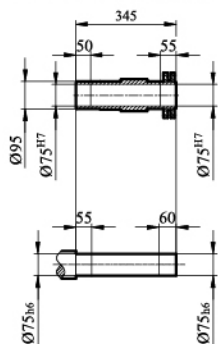
FH/ FHZ/ FHF97输出轴
