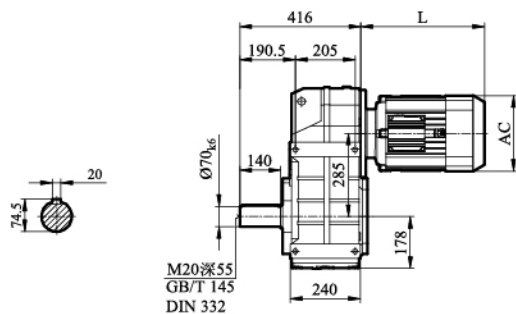
FA/ FH/ FV97
