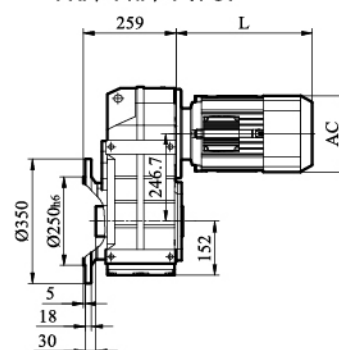
FAF/ FHF/ FVF87
