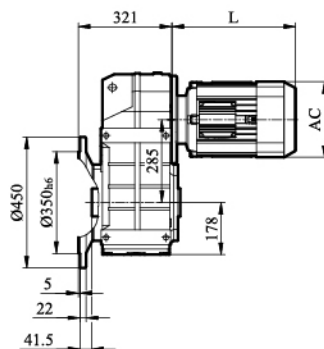
FH/ FHZ/ FHF97输出轴
