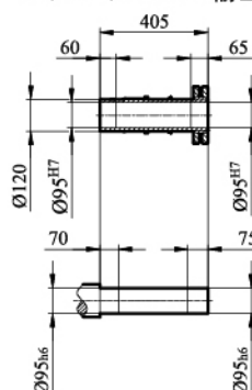
FH/ FHZ/ FHF107输出轴
