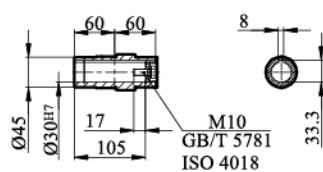
FA/ FAZ/ FAF37输出轴
