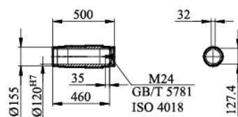
FA/ FAZ/ FAF157输出轴
