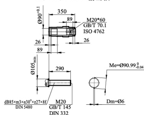
FV/ FVZ/ FVF107输出轴
