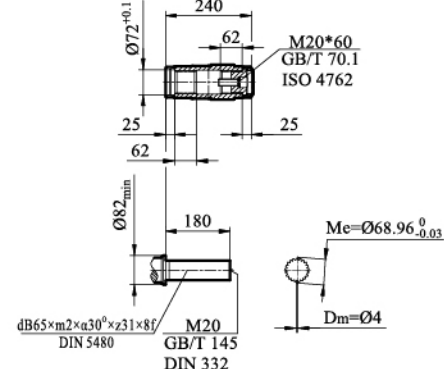
FV/ FVZ/ FVF87输出轴
