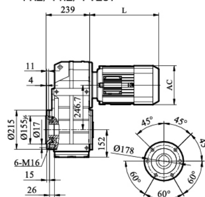
FAZ/ FHZ/ FVZ87
