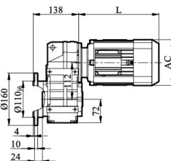
FAF/ FHF/ FVF37
