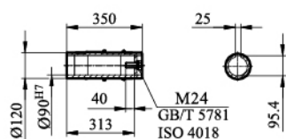
FA/ FAZ/ FAF107输出轴
