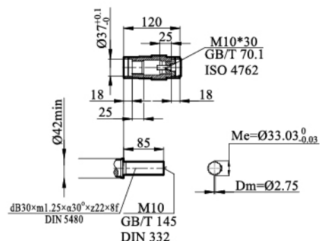
FV/ FVZ/ FVF37输出轴
