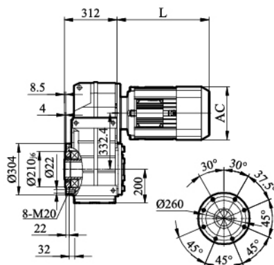
FAF/ FHF/ FVF107
