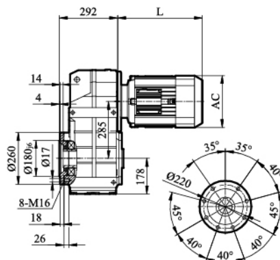
FAF/ FHF/ FVF97
