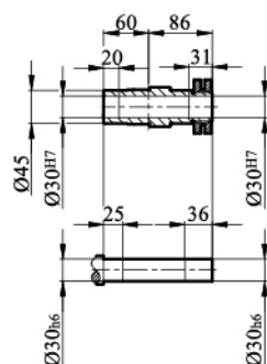
FH/ FHZ/ FHF37输出轴
