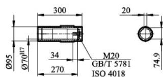
FA/ FAZ/ FAF97输出轴
