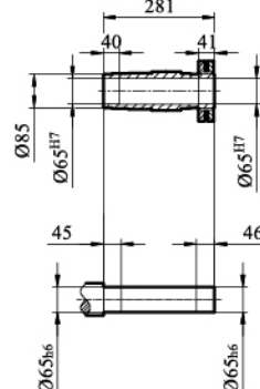
FH/ FHZ/ FHF87输出轴
