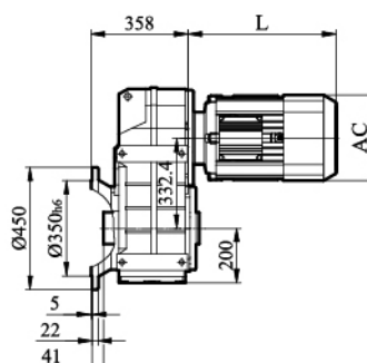
FAF/ FHF/ FVF107
