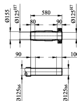
FH/ FHZ/ FHF157输出轴
