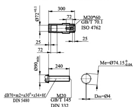
FV/ FVZ/ FVF97输出轴
