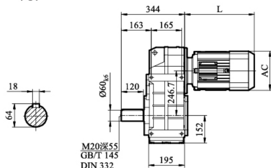
FA/ FH/ FV87
