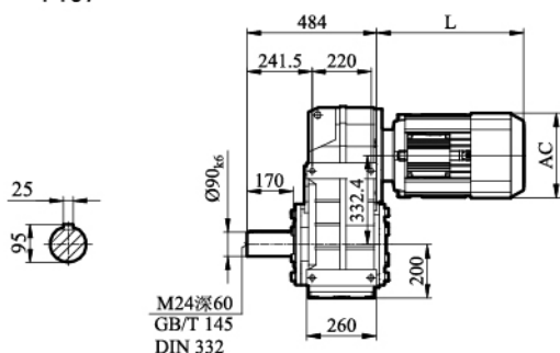
FA/ FH/ FV107
