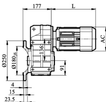
FH/FHZ/FHF57输出轴
