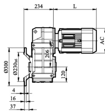
FH/FHZ/FHF77输出轴
