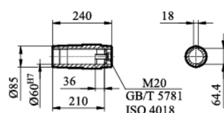
FA/ FAZ/ FAF87输出轴
