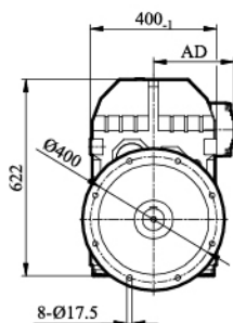
FV/ FVZ/ FVF97输出轴
